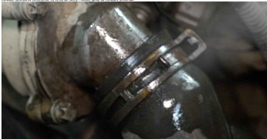
16 Săbiți clemele furtunurilor lichidului de răcire. Folosiți clești pentru coliere Click-R.
