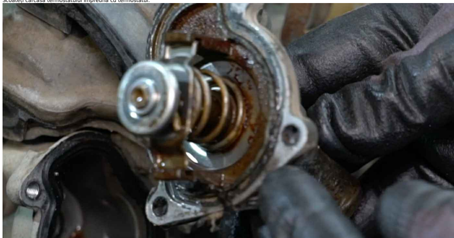
22 Acoperiți locul de montare al carcasei termostatului cu o cârpă din microfibră pentru a preveni pătrunderea murdăriei și a obiectelor străine în sistem.
