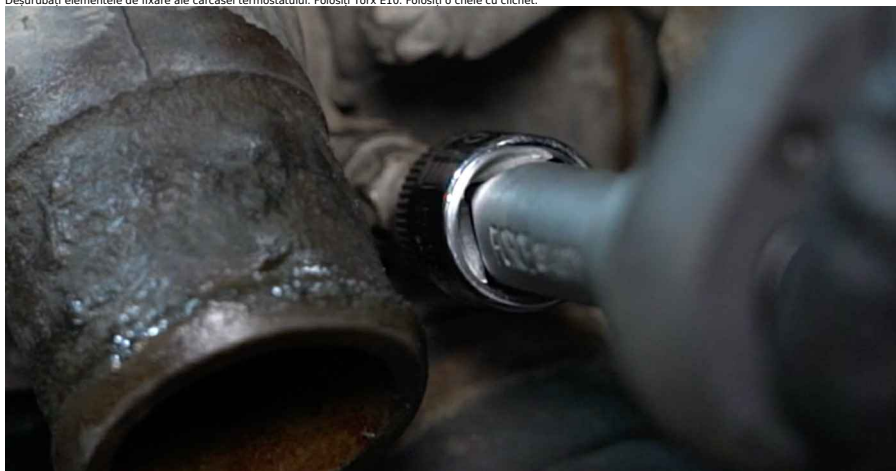
21 Scoateți carcasa termostatului împreună cu termostatul.
